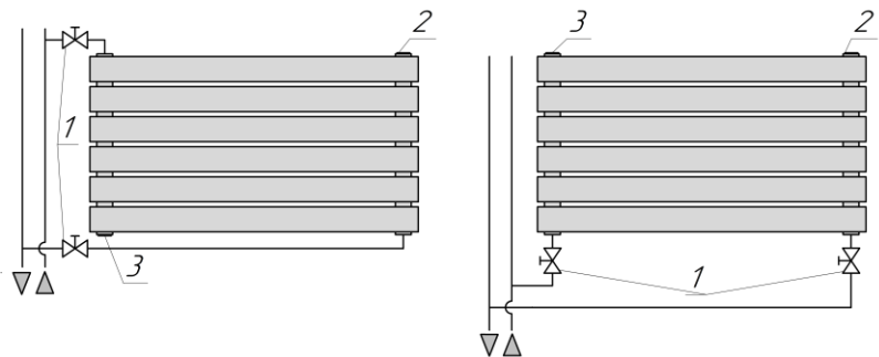
Рис. 3. 1. Вентиль (кран). 2. Кран Маевского-воздухоотводчик. 3. Пробка глухая.
