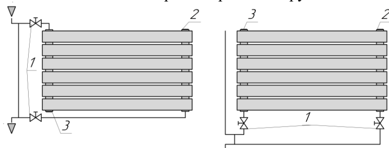
Рис. 2. 1. Вентиль (кран). 2. Кран Маевского-воздухоотводчик. 3. Пробка глухая.
